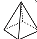
Piramid
