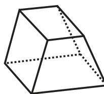
Trapeziod
