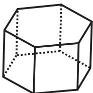
Prisma Heksagon
