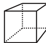
Kiub
