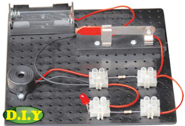
( Reka Bentuk dan Teknologi ) 制作发光二极管与蜂鸣器电路 (神奇的电子世界) 5cm — 电与电子 ELEKTRIK & ELEKTRONIK
