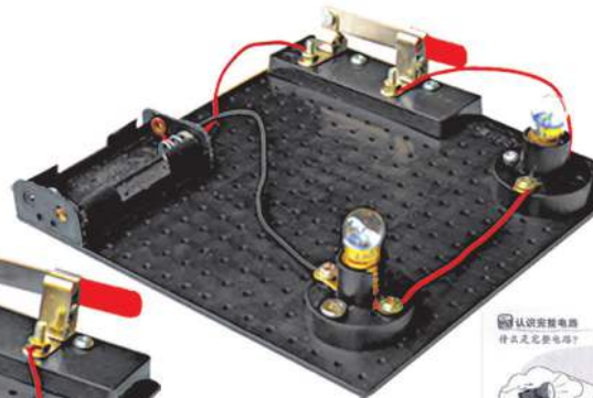
B Kaedah 2 并联电路
