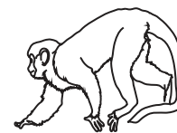
Monyet
