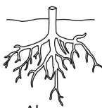
Akar Tunjang
