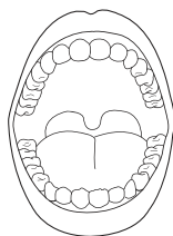
Gigi Kekal
